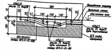
РАЗРЕЗ 1-1
