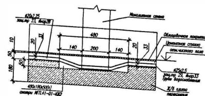
РАЗРЕЗ 2-2
